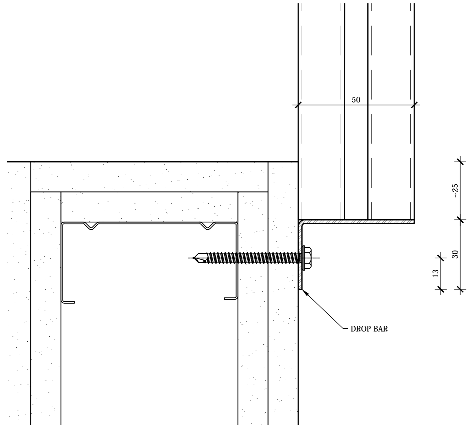
WINDOW SILL BOTTOM BAR DETAIL 3 SCALE: 1:1 @ A2
